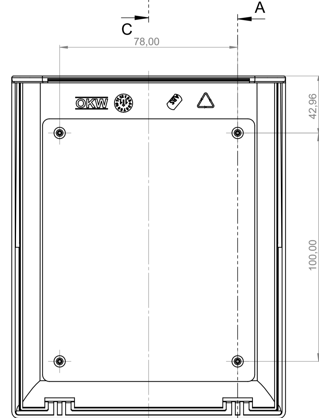
Oberteil Innenansicht Top, real inside view
