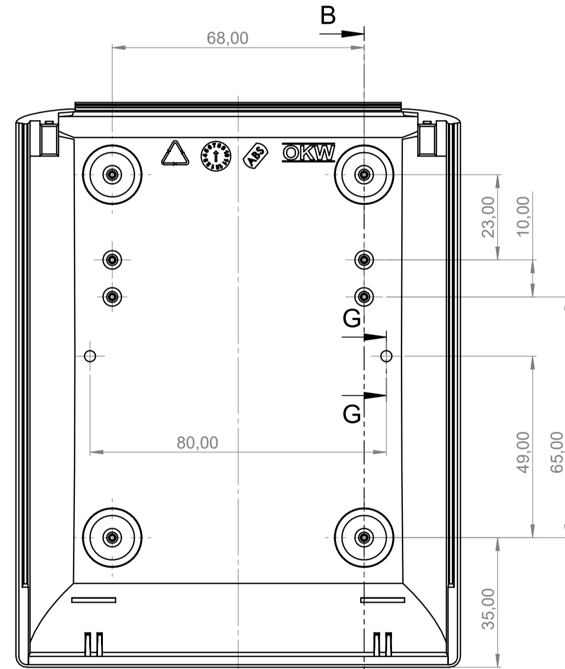
Unterteil Innenansicht Base, real inside view
