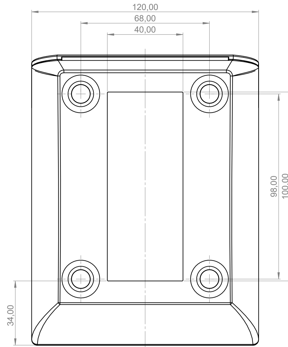
Unterteil Untersicht Base, real outside view
