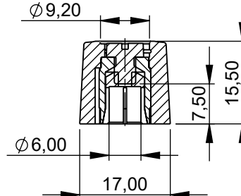
Schnitt A-A
