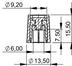
Schnitt B-B
